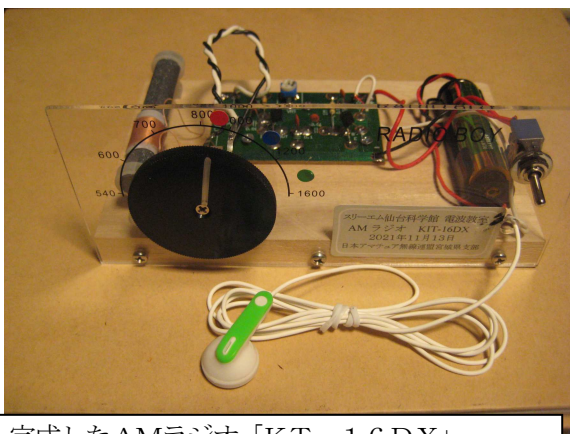
完成したAMラジオ「KT-16DX」
